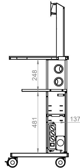
SEZ A-A
