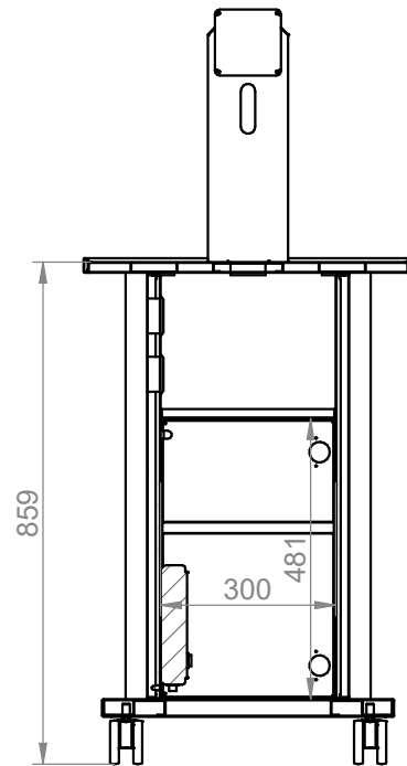
SEZ B-B
